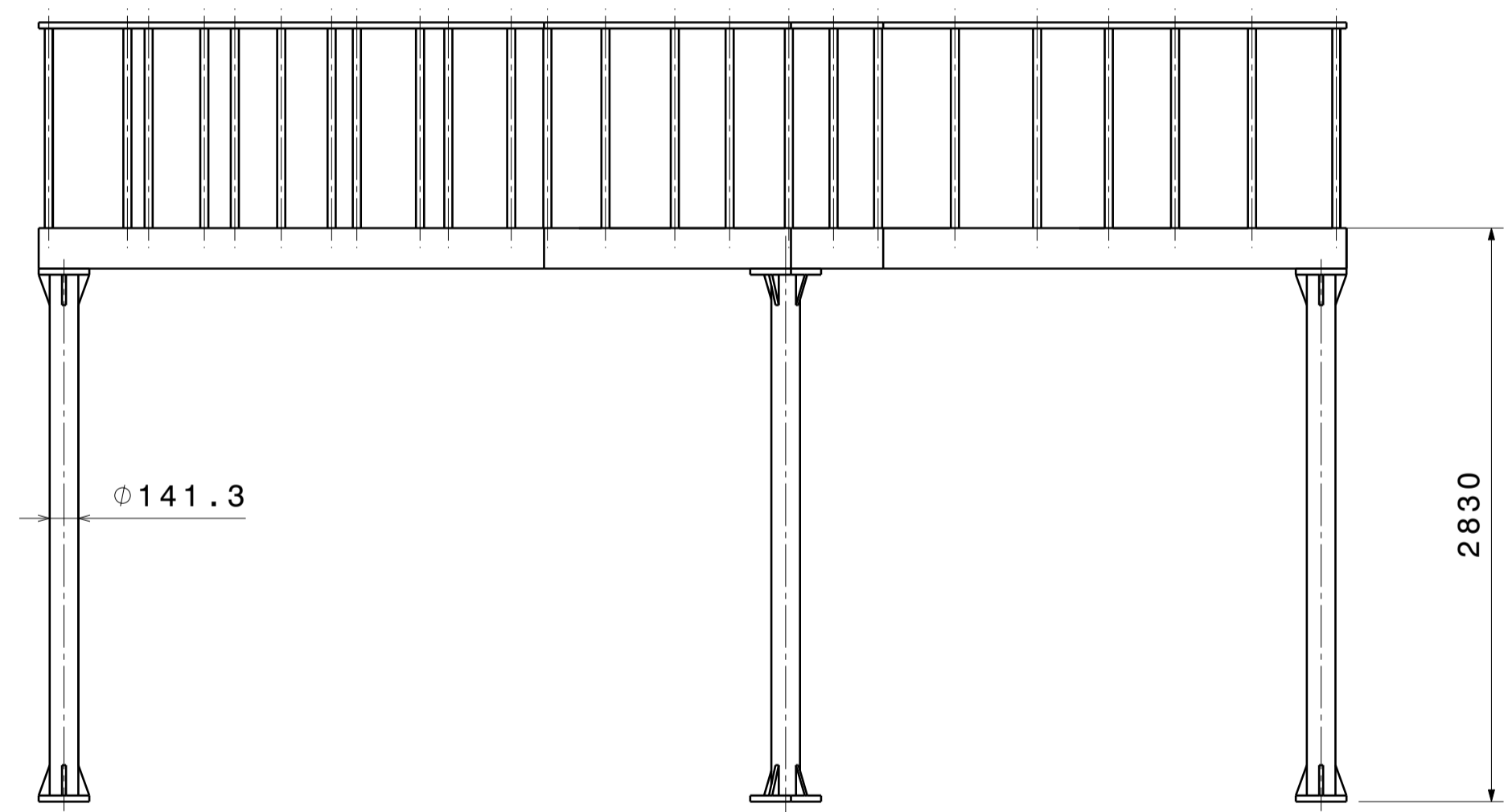
Front view Scale: 1:30
