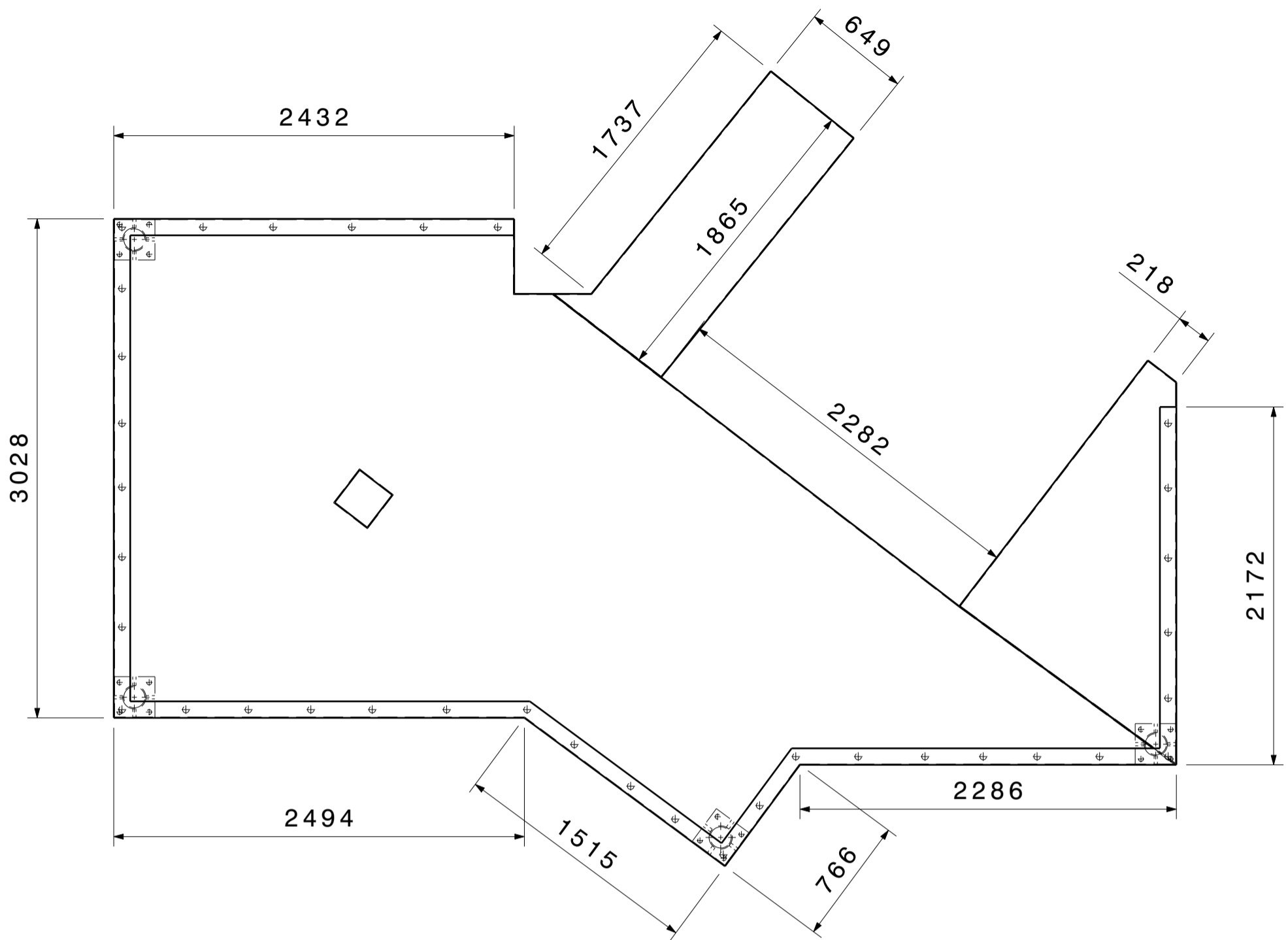
Top view Scale: 1:30
