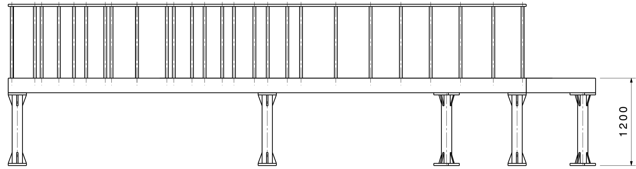
Front view Scale: 1:30
